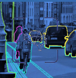
Neural Dedektör
