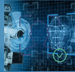
Yüz Tanıma
