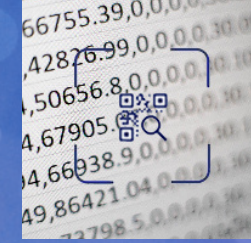
QR/Barkod Okuma
